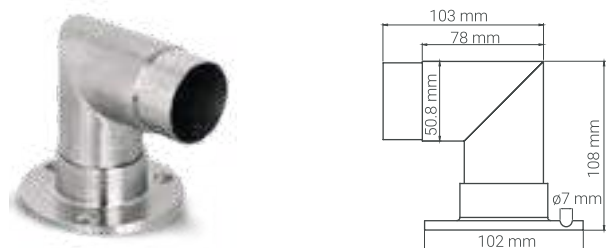
Curva 90° recta brida
