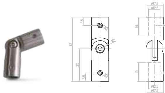
Niple articulado p/unión de barra
