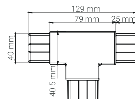
Empalme tee tubo cuadrado exterior
