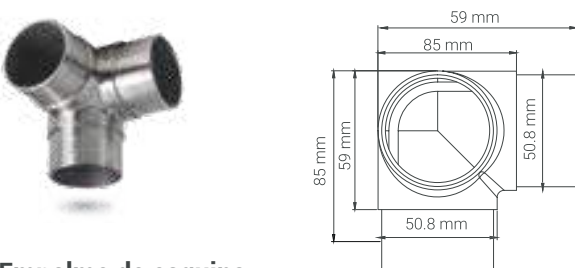
Empalme de esquina
