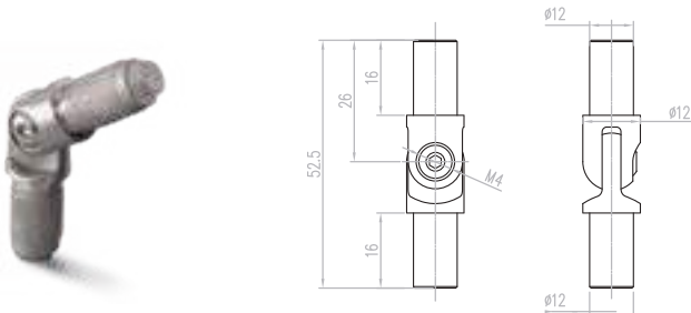
Niple articulado p/unión de tubo
