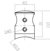
Soporte para barra pasante
