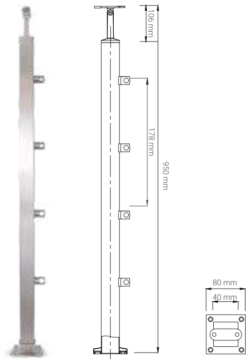
Balaustre cuadrado para tubo o barra Ø 12mm
