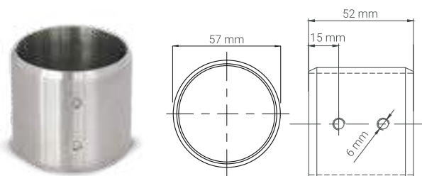
Empalme tubo exterior
