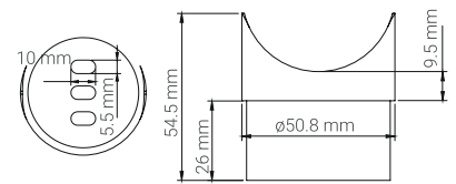
Soporte tubo boca de pescado
