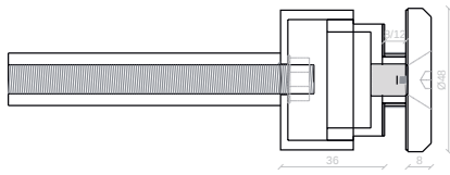
Botón distanciador chico alto
