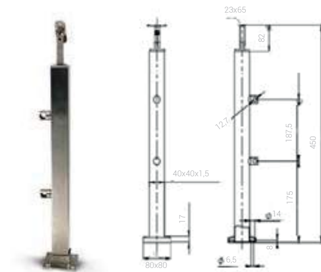
Balaustre cuadrado corto para tubo o barra Ø 12mm
