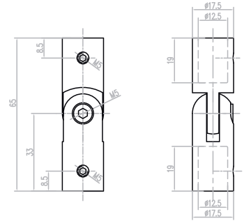
Niple articulado p/unión de barra
