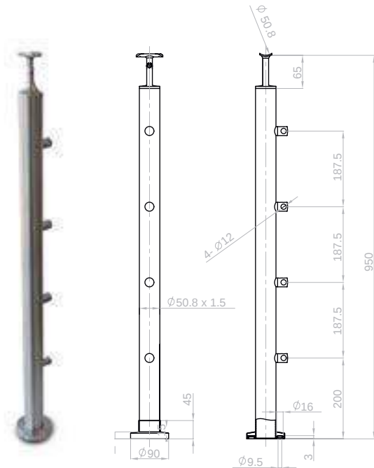
Balaustre redondo para tubo o barra Ø 12mm
