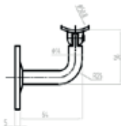
Soporte barra pasamanos articulado
