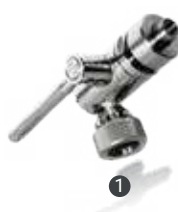
Grifos de nivel 1 Superior: \varnothing 1/2" R/W 2 Inferior c/purga esférico: \varnothing 1/2" R/W
